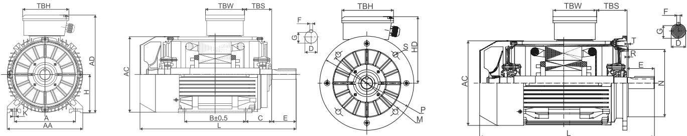
IM B5 - D Flange
